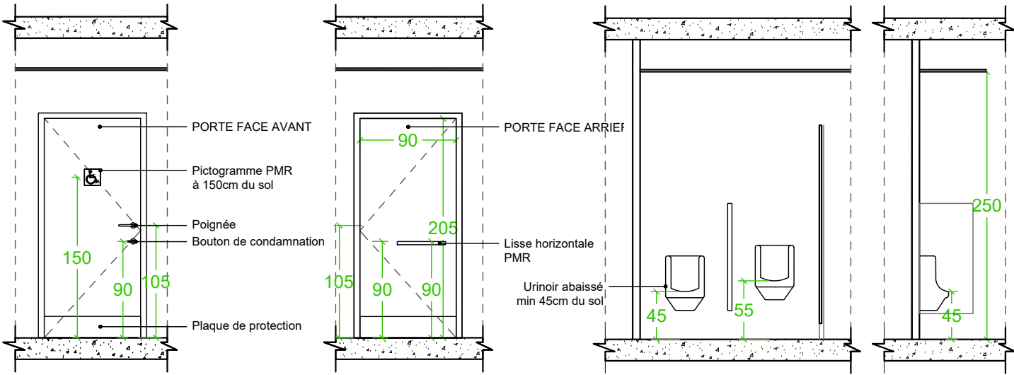
Détails sanitaire PMR Hommes / Femmes - Ech: 1:50
