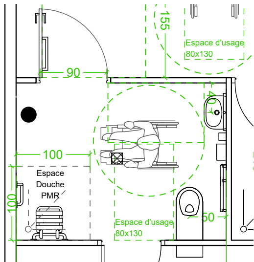
Plan sanitaire PMR Hommes - Ech: 1:50
