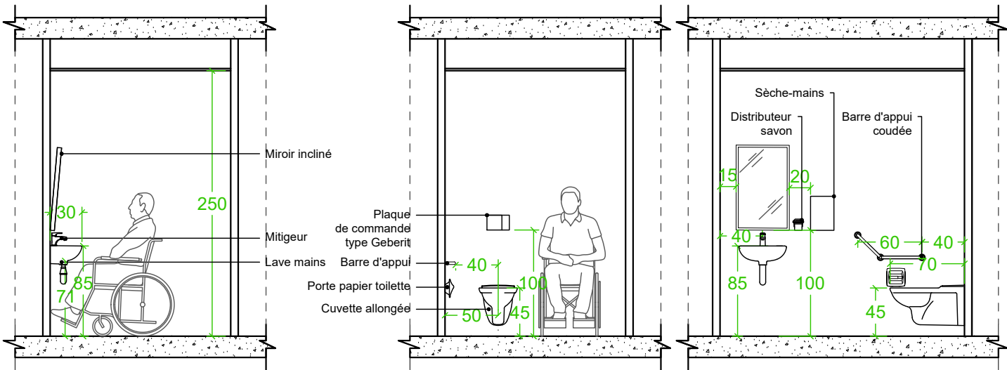
Détails vasque sanitaires - Ech: 1:50
