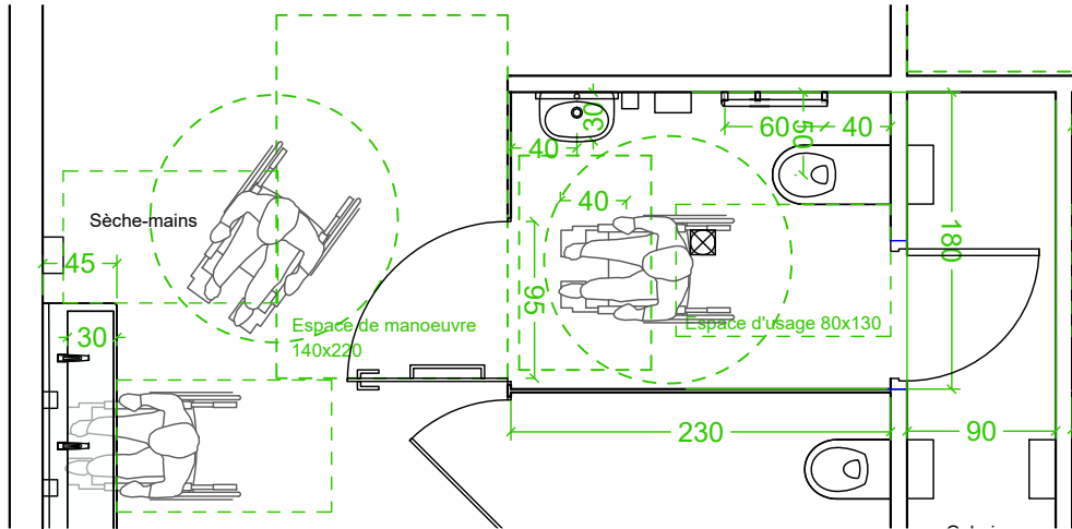
Plan sanitaire PMR Hommes - Ech: 1:50
