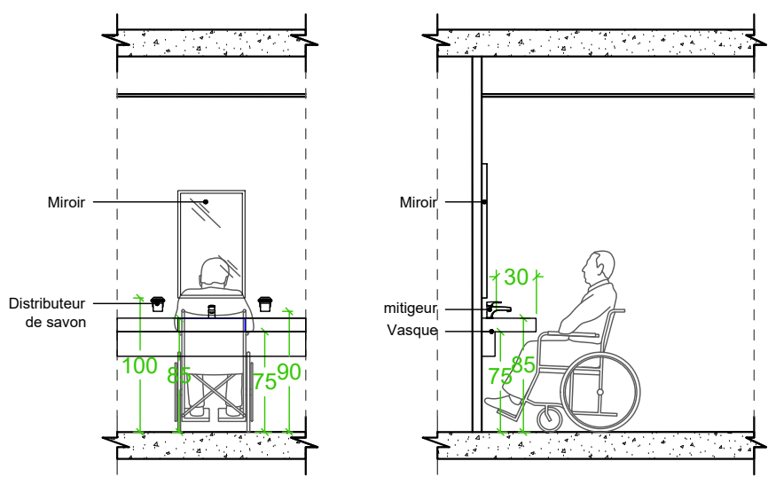
Détails vasque PMR sanitaires - Ech: 1:50
