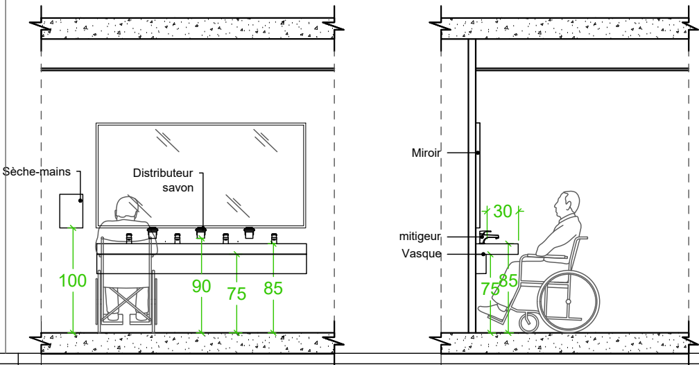
Détails vasque sanitaires - Ech: 1:50
