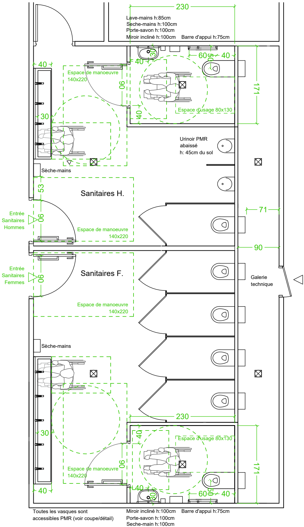
Plan sanitaires C.4 - Ech: 1:50
