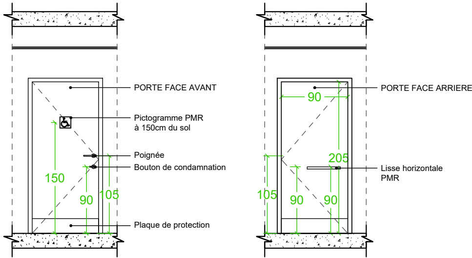
Plan sanitaire PMR Hommes - Ech: 1:50
