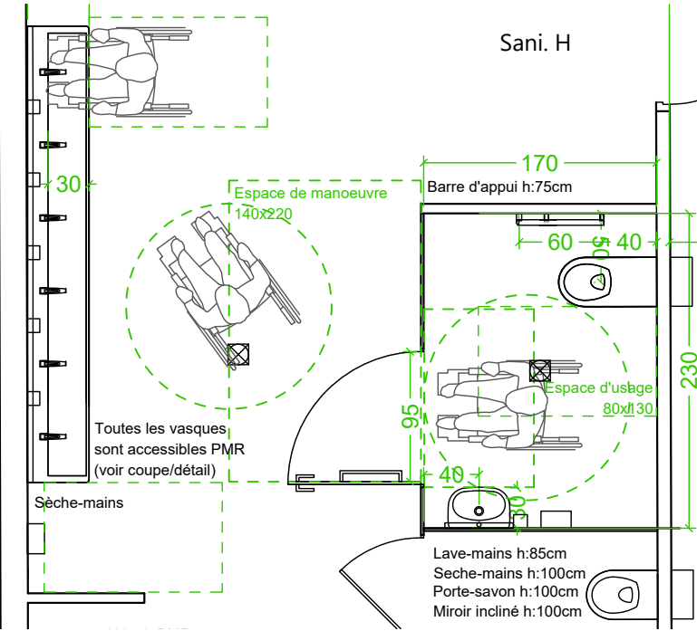
Plan sanitaires C.8 - Ech: 1:50
