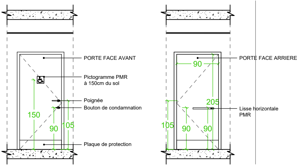
Détails Porte entrée sanitaires - Ech: 1:50
