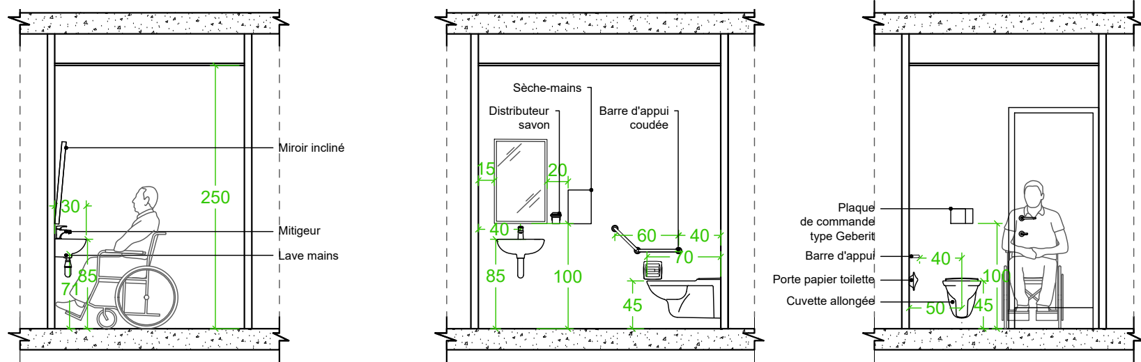
Détails sanitaire PMR Hommes / Femmes - Ech: 1:50
