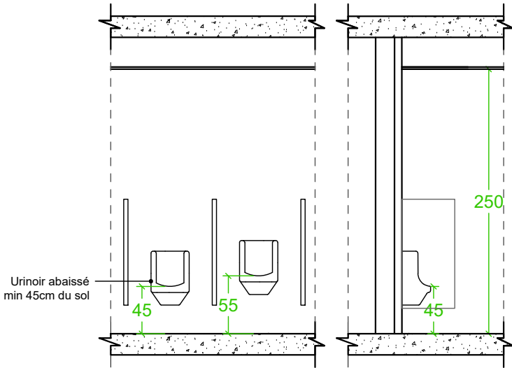
Détails urinoirs sanitaires - Ech: 1:50
